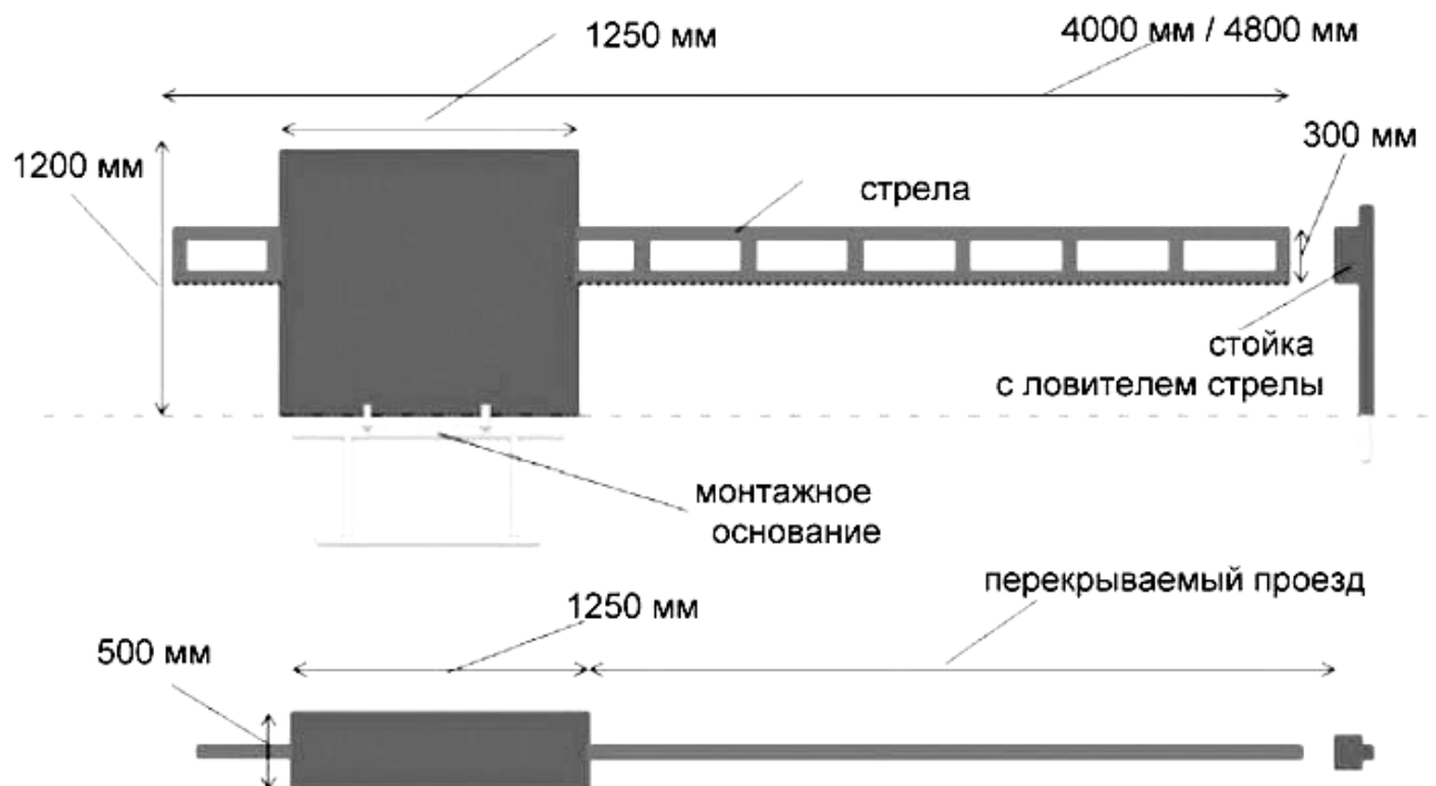
Рис.2 Размеры шлагбаума откатного
